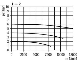
Durchflussdiagramm
